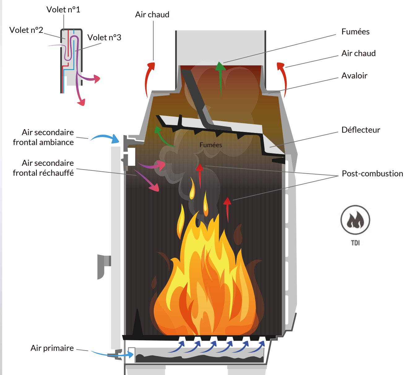
SCHÉMA DE LA BI-COMBUSTION
